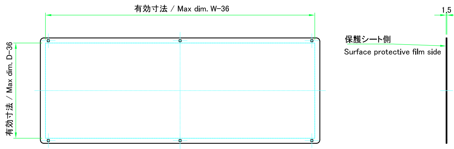
パネル表面 / Panel Frontside
