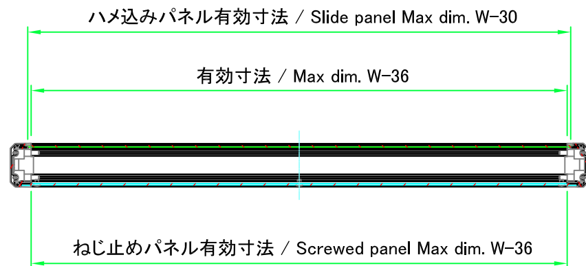
A-A ( 1 : 4.5 )
